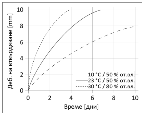
Диаграма 1: Скорост на втвърдяване на SikaTack® Panel-50
