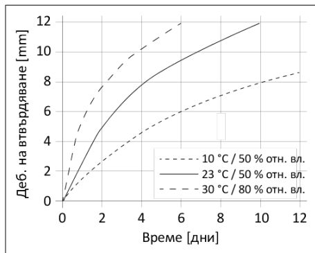
Диаграма 1: Скорост на втвърдяване на SikaTack® Panel
